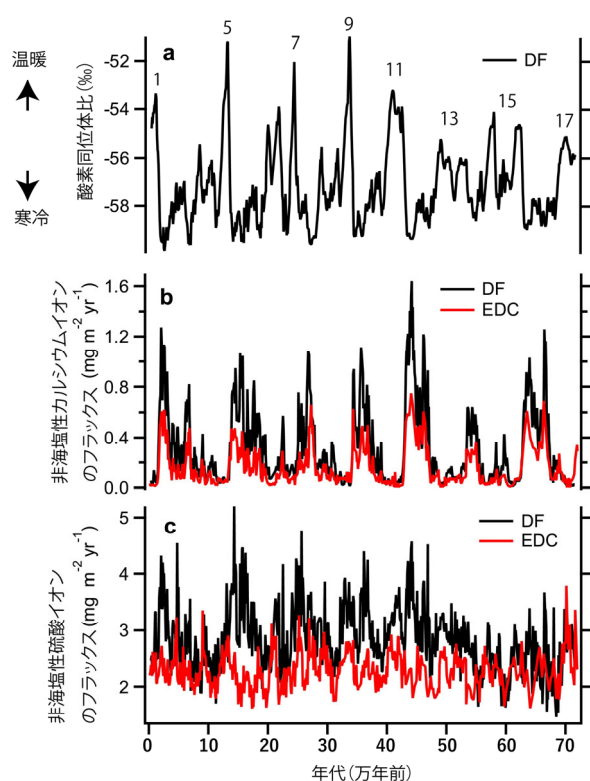
図3：過去72万年間を通じてのドームふじコアの酸素同位体比、および非海塩性カルシウムイオンと非海塩性硫酸イオンのフラックスの変動。ドームふじコア（DF）との比較のためにドームCコア（EDC）のデータも示す。酸素同位体比は気温変動の指標で、値が大きいほど温暖だったことを意味する。aに番号で示したのは、海底堆積物から決められた酸素同位体ステージであるが、ここでは間氷期のみに番号をつけた。非海塩性カルシウムイオンは、カルシウムイオンの総量から海塩起源のものを差し引いたもので、鉱物ダストの指標とされる。
