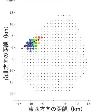
図4：2023年5月27日にテレスコープアレイ実験で検出された極めて高いエネルギー宇宙線の信号（画像提供：大阪公立大学）
