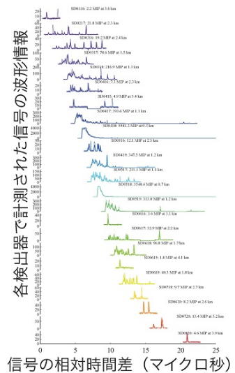
図4：2023年5月27日にテレスコープアレイ実験で検出された極めて高いエネルギー宇宙線の信号（画像提供：大阪公立大学）
