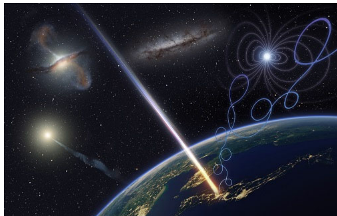
図2：極高エネルギー宇宙線による次世代天文学の概念図。極高エネルギー宇宙線は宇宙磁場内をほぼ直進するため、その到来方向が起源方向を指し示すと期待されている。背景には宇宙線起源の候補天体である活動銀河核や強磁場中性子星を表している (画像提供：大阪公立大学/京都大学/Ryuunosuke Takeshige)
