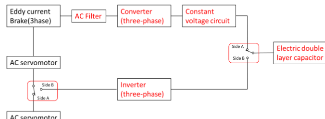
蓄積・回生システムの構成
