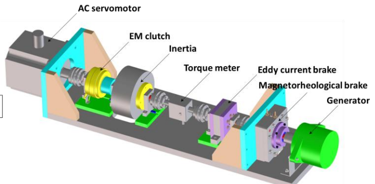
ブレーキエネルギーの蓄積・回生システムの実験機
