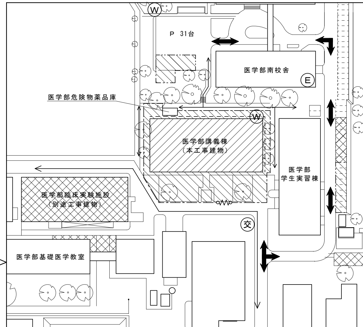
本工事建物配置図 S = 1 / 1000
