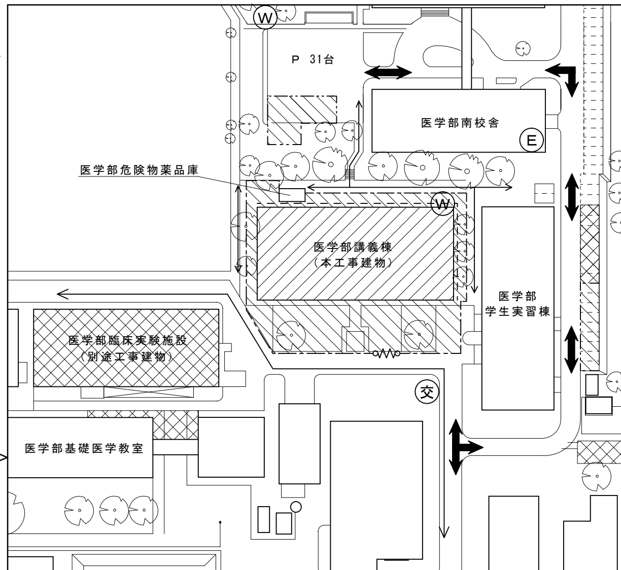
本工事建物配置図 S = 1 / 1000
