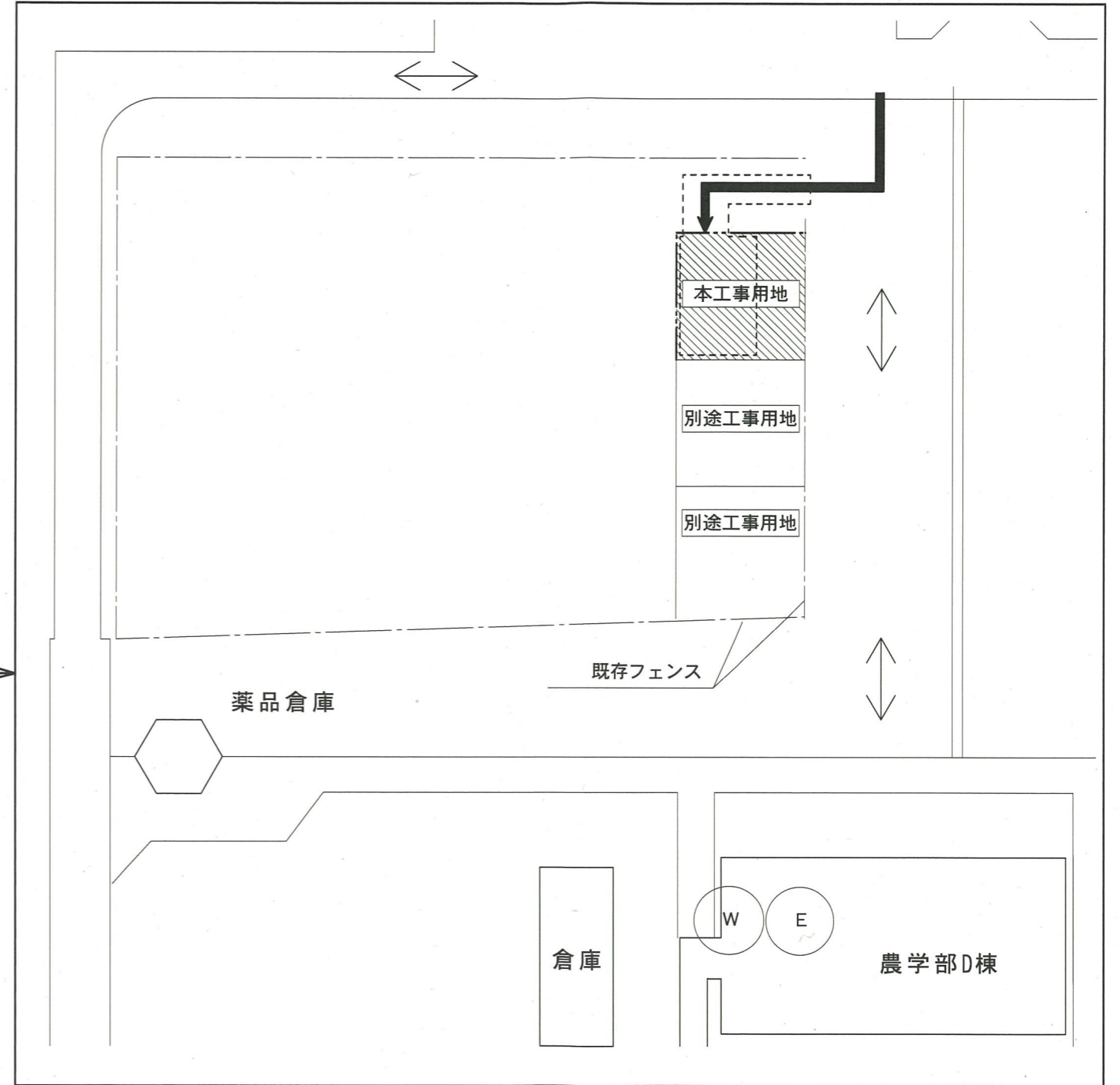
本工事用地配置図 S=1/500
