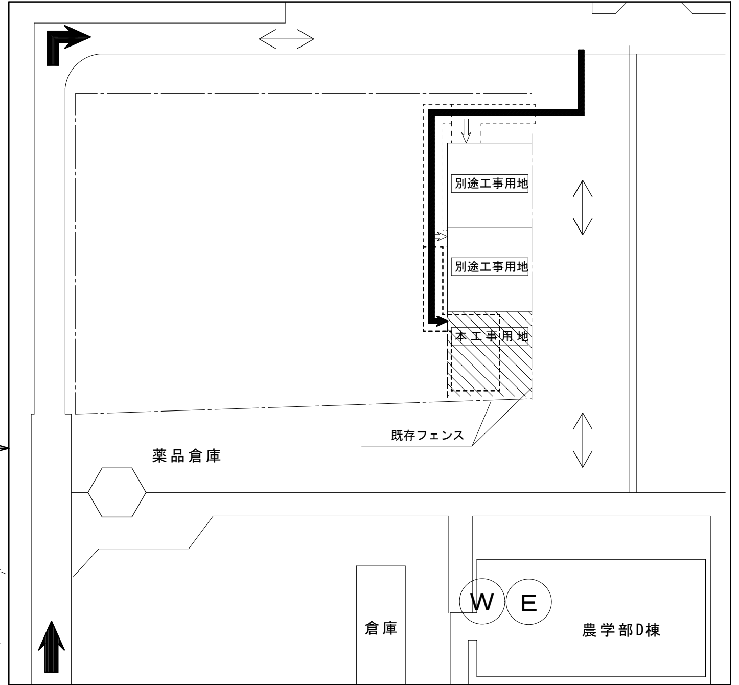
本工事用地配置図 S=1/500
