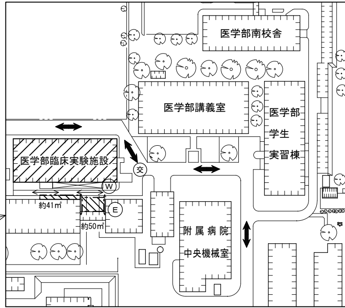
工事用地② 配置図 S = 1 / 1200
