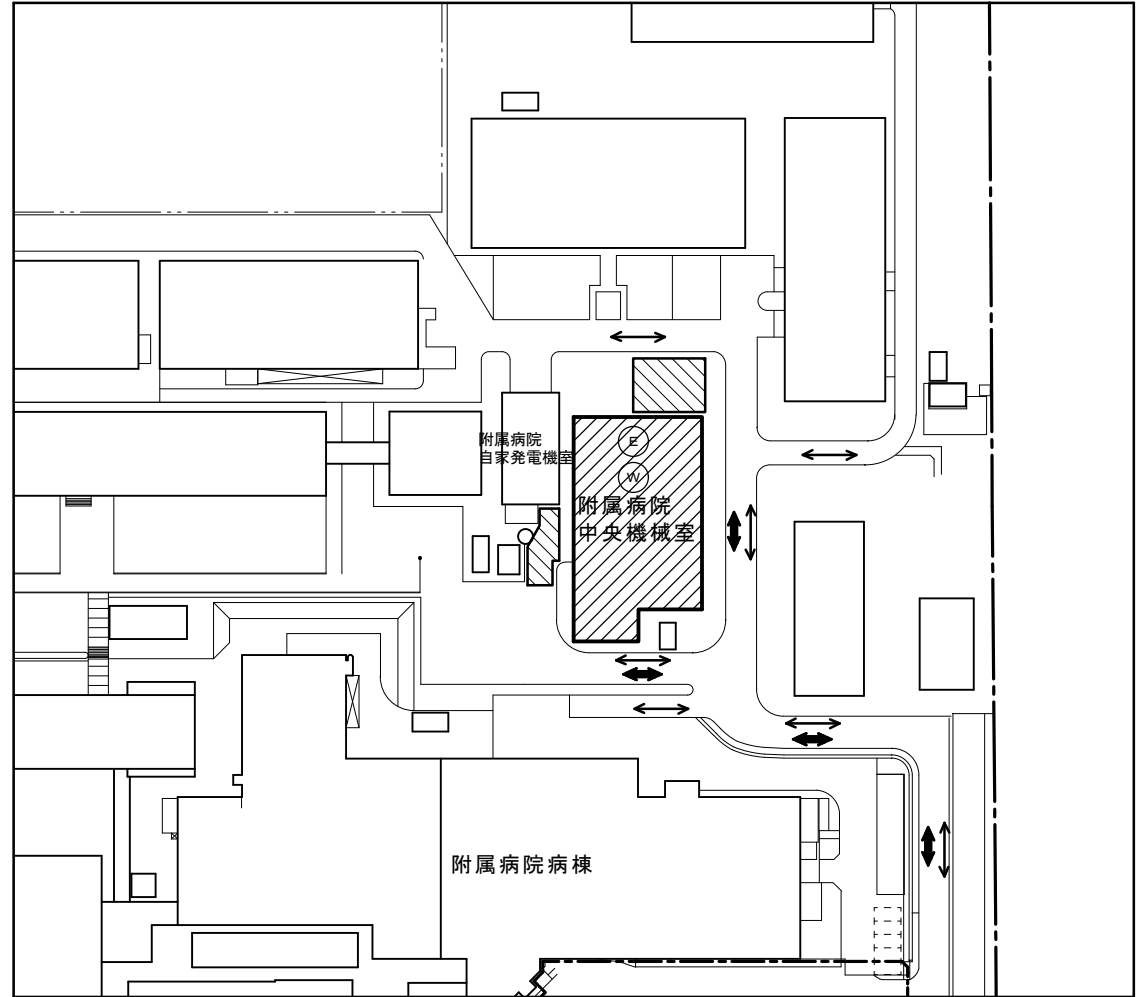
本工事建物周辺 配置図 S = 1 / 1000
