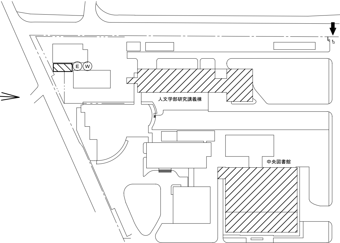
本工事建物周辺 配置図 NoScale
