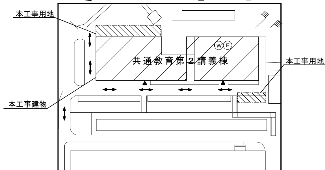
本工事建物周辺 配置図 S = 1 / 600
