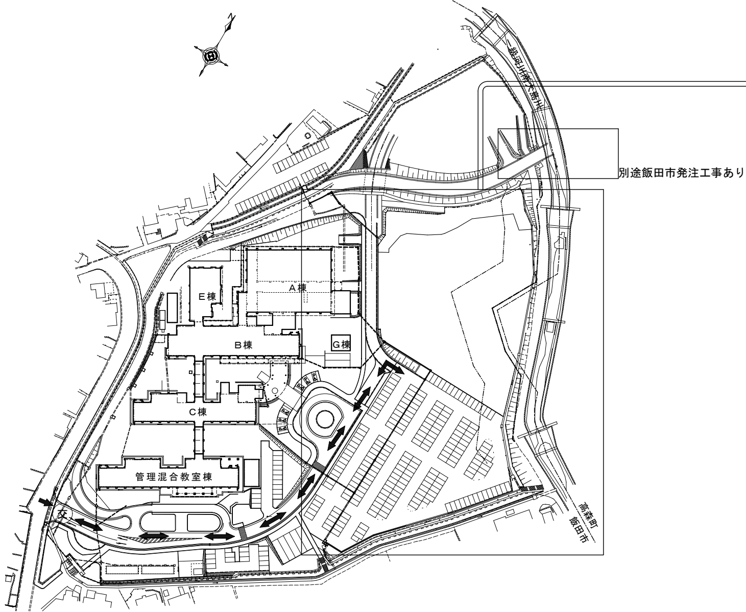
飯田市エス・バード配置図 S = 1 / 2 0 0 0
