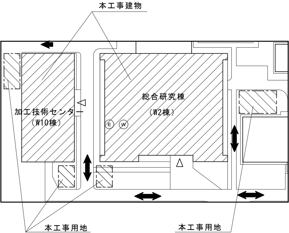
本工事用地 配置図 S=1/500
