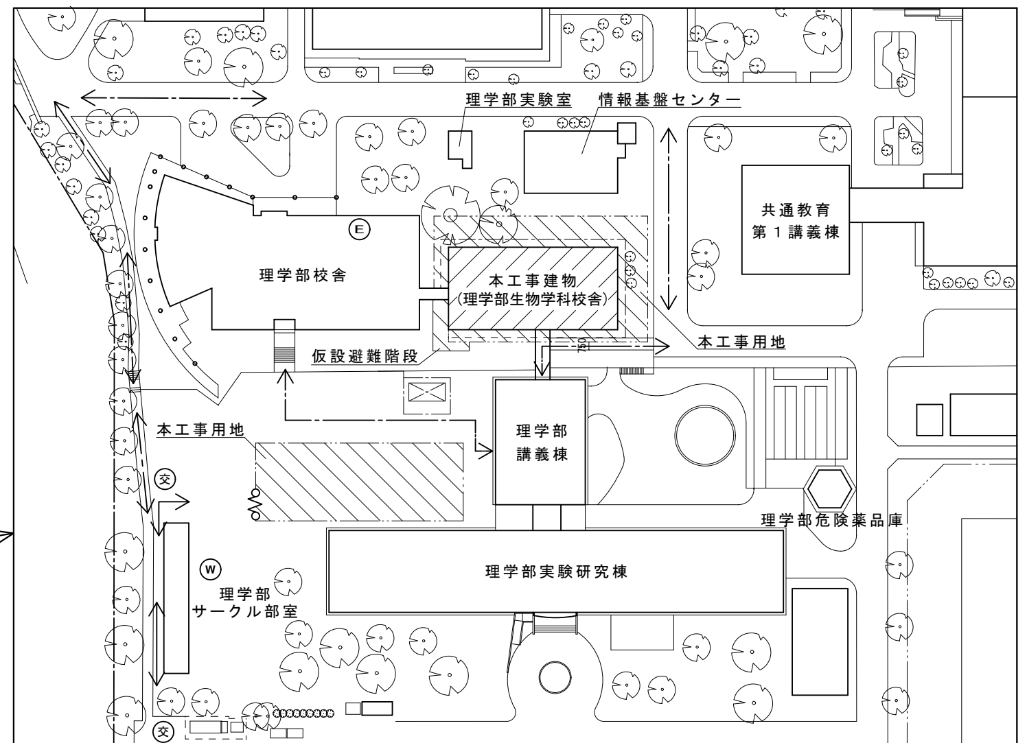
本工事建物周辺 配置図 S=1/1000
