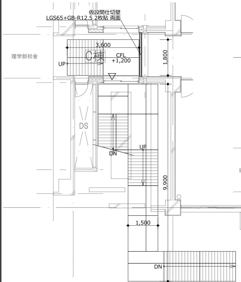
仮設避難階段 1階平面図 (参考図)
