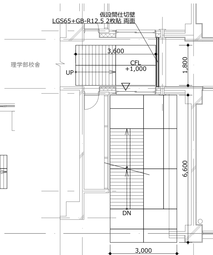
仮設避難階段 2~5階平面図 (参考図)
