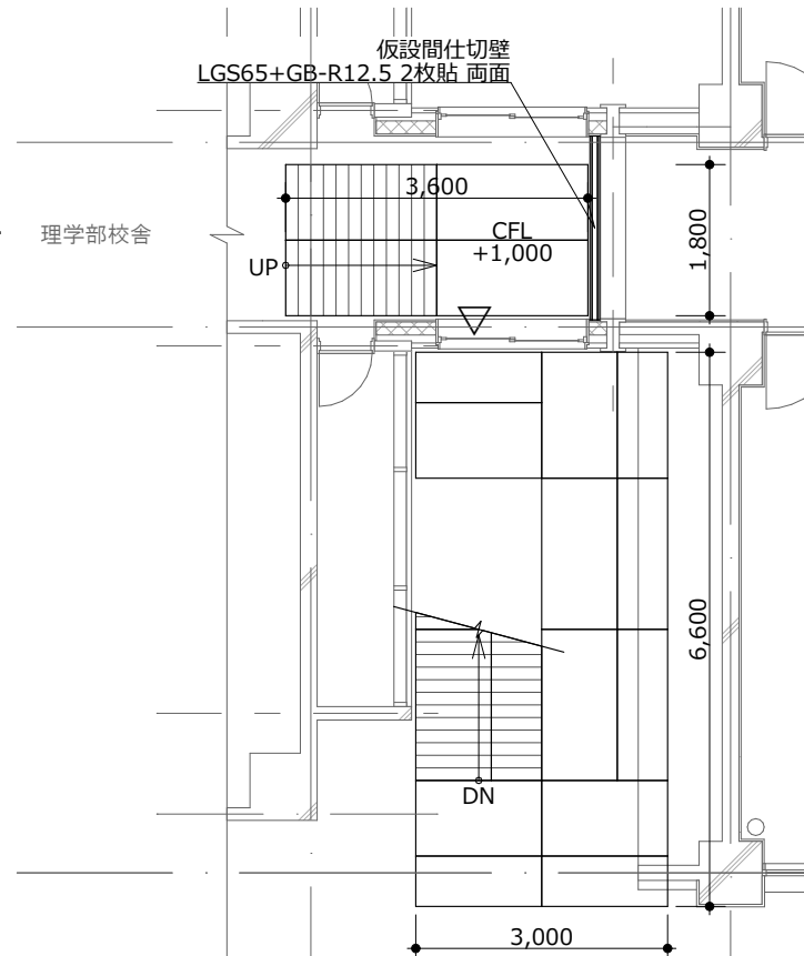
仮設避難階段 6階平面図 (参考図)
