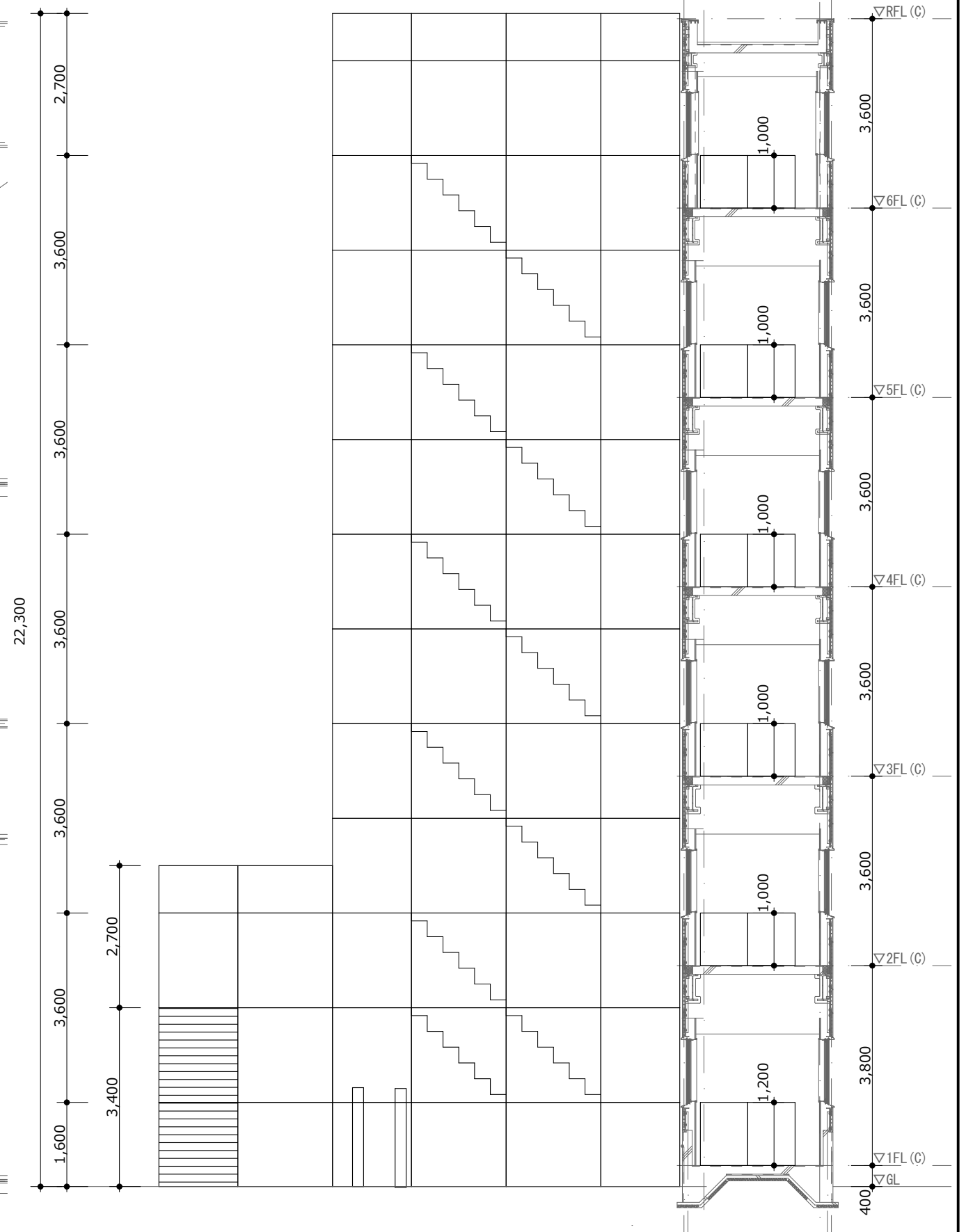
仮設避難階段 東立面図・渡り廊下断面図 S=1/100
