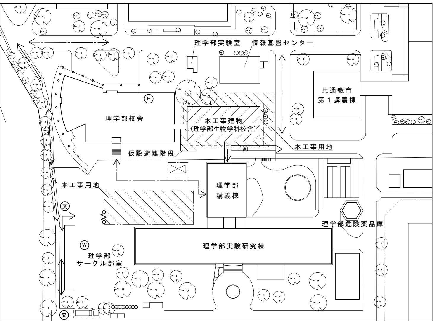
本工事建物周辺 配置図 S=1/1000
