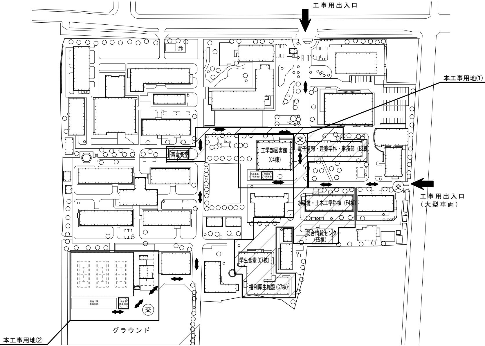
長野（工学）キャンパス 配置図 S = 1 / 2 0 0 0
