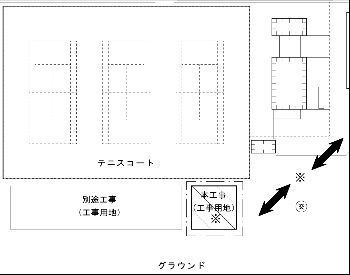
本工事用地 配置図 S = 1 / 5 0 0
