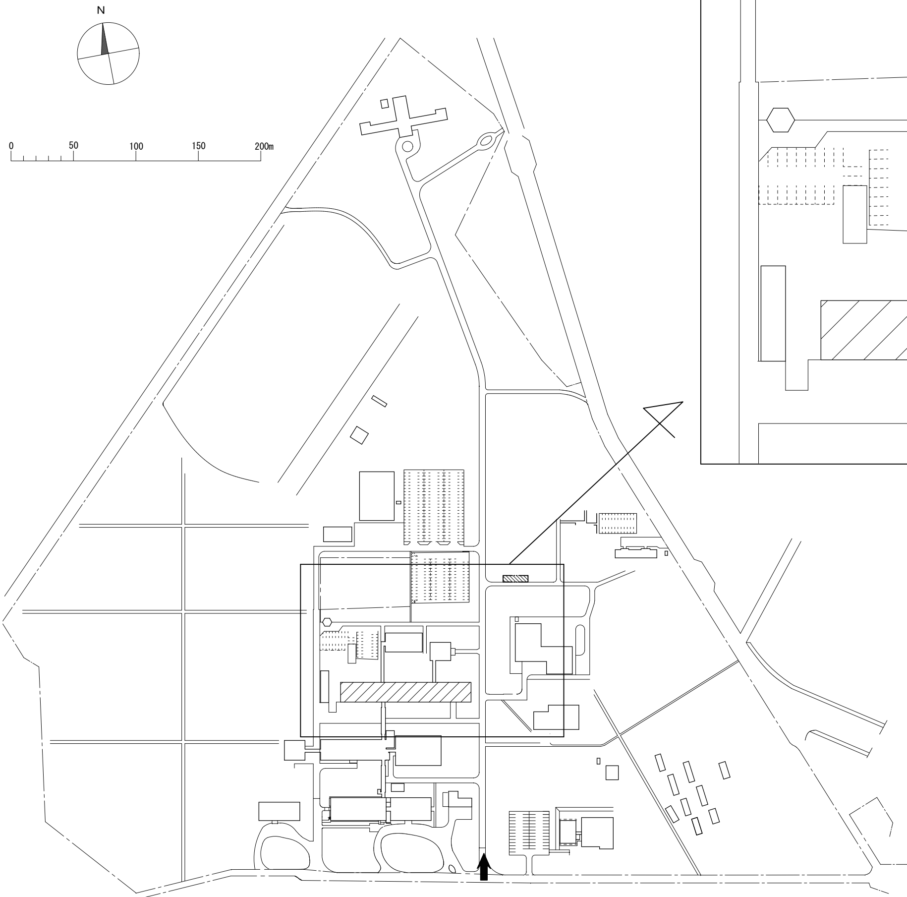
伊那キャンパス配置図 S = 1/3000
