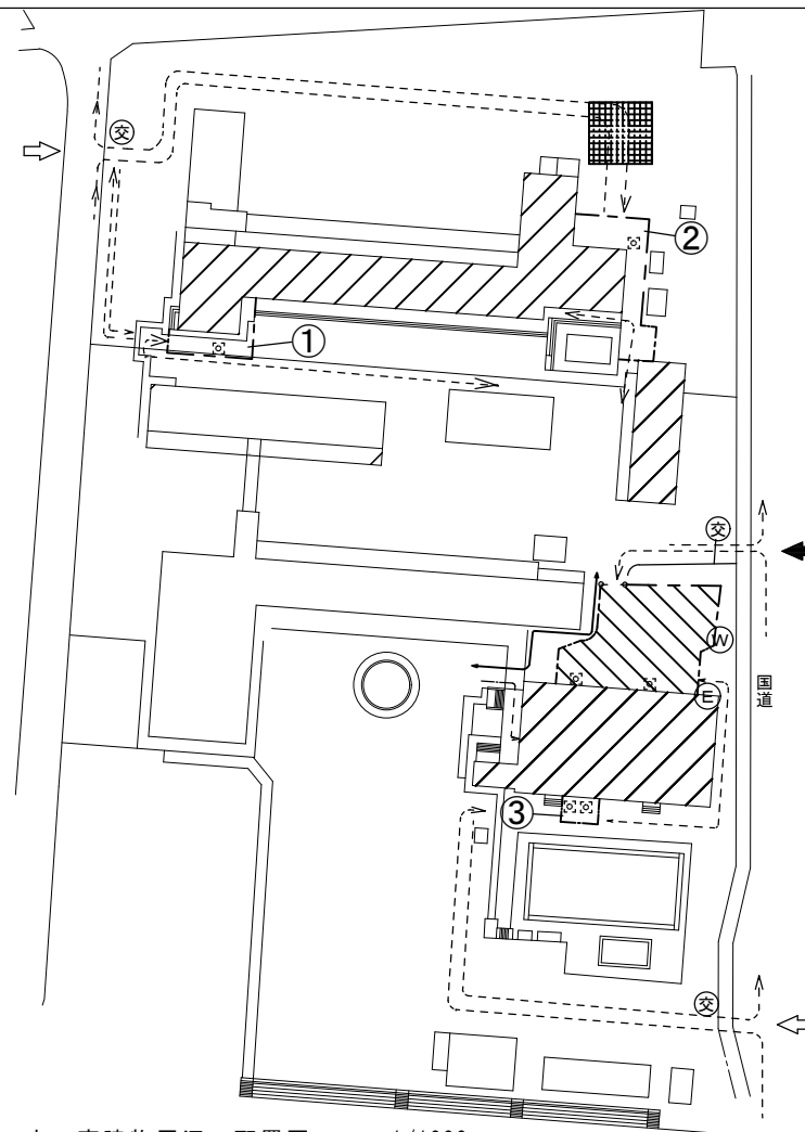
本工程建物周辺 配置図 S = 1/1000
