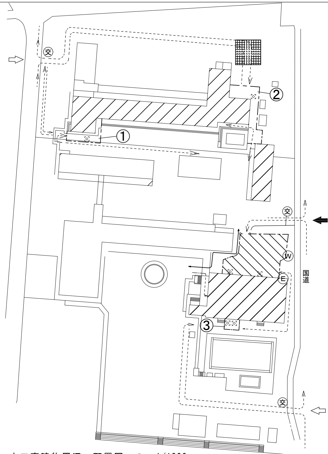
本工事建物周辺 配置図 S = 1/1000
