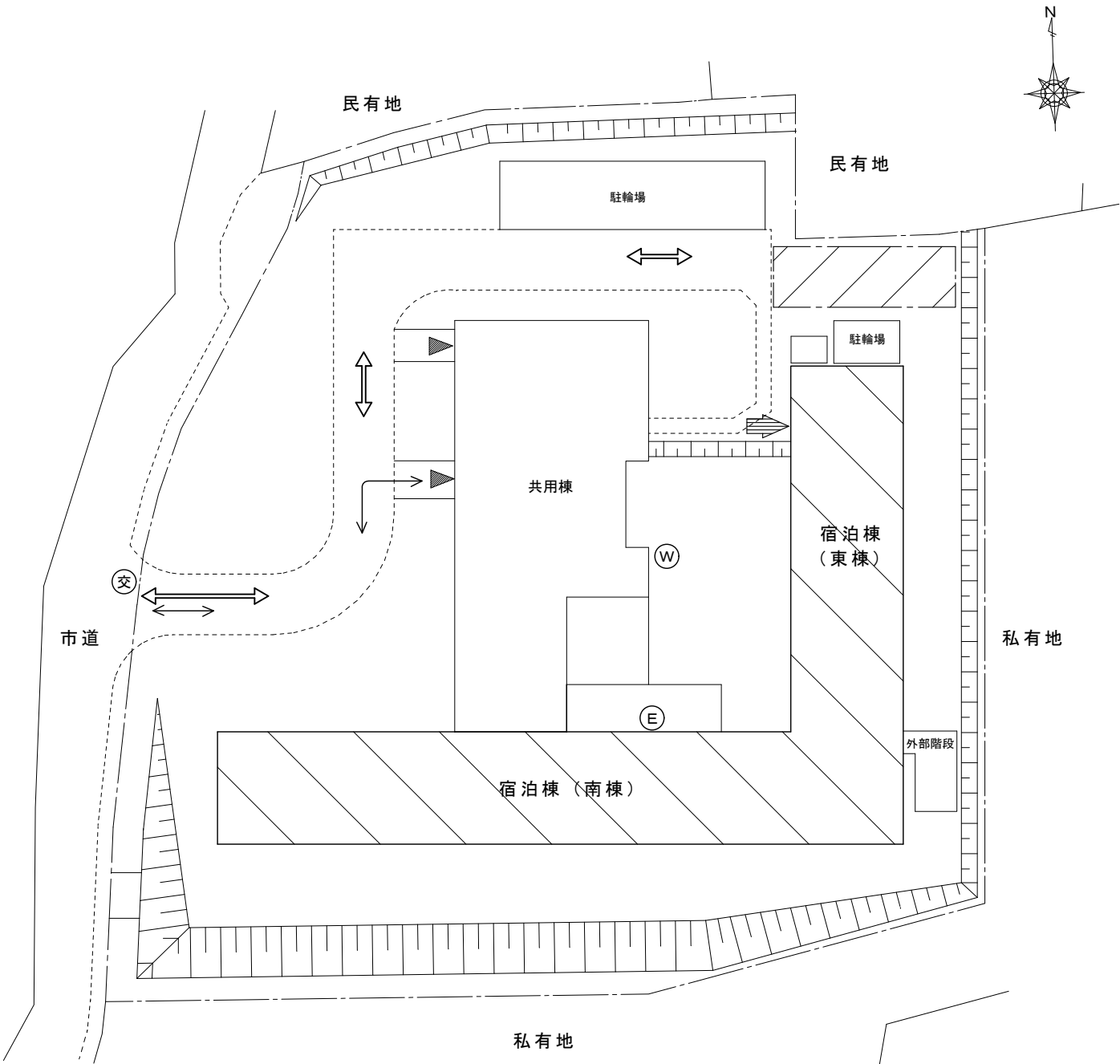
本工事建物周辺配置図 S=1/400
