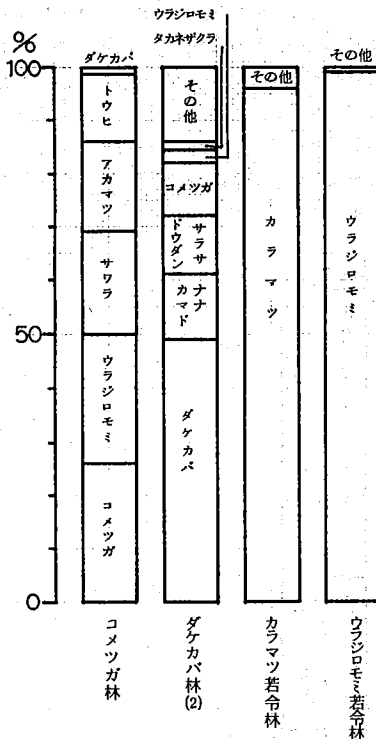
図4. 各群落の相対基底面積 (RBA%)
