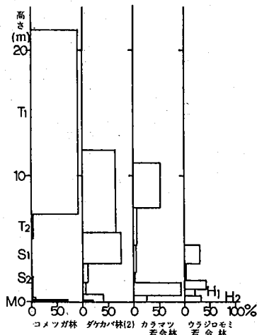
図2. 各群落の階層構造。横軸は植被率(%)
