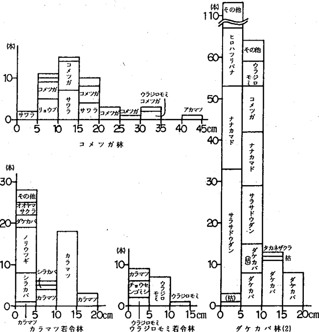
図3. 各群落(森林のみ)の胸高直径(DBH)ヒストグラム
