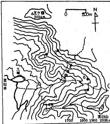
図1. 美ヶ原南斜面の地形図と調査区(1～6)
