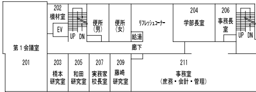
2 階
