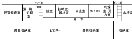
東御市大室農場1階平面図
