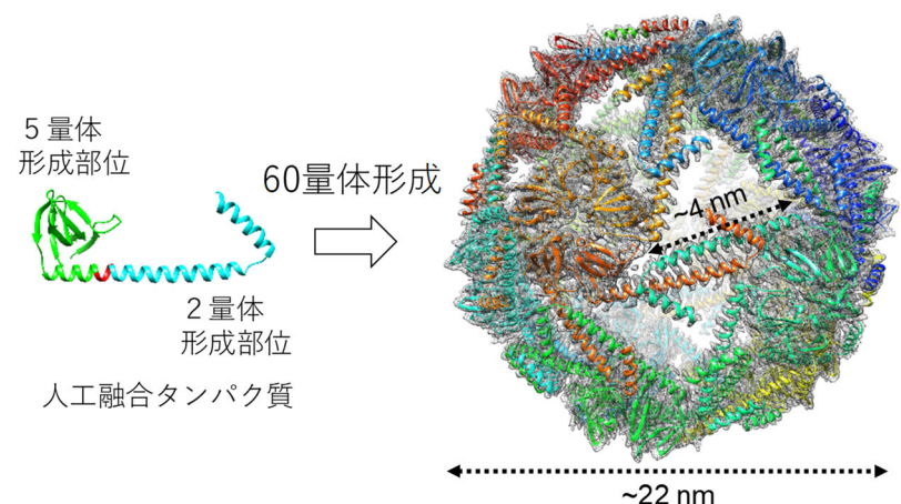
図2 クライオ電子顕微鏡単粒子解析によって得られたタンパク質ナノ粒子TIP60の立体構造
