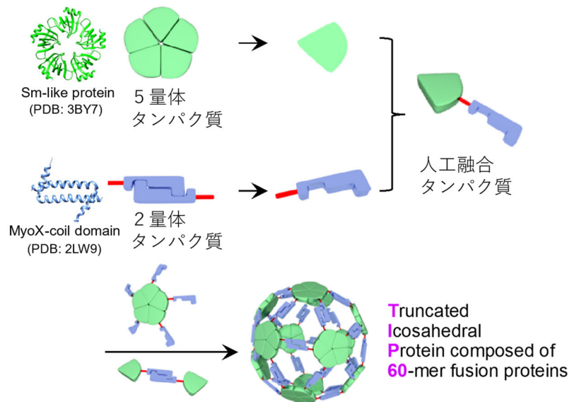
図1 人工融合タンパク質の設計とタンパク質ナノ粒子TIP60の形成 5量体タンパク質と2量体タンパク質を連結した人工融合タンパク質同士が60個自発的に組み上がってTIP60が形成される。
