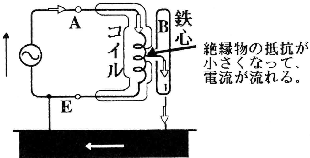
図 3.3 漏電の状態
