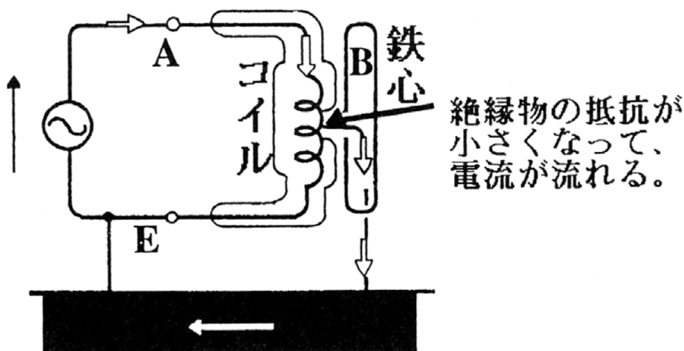
図 3.3 漏電の状態
