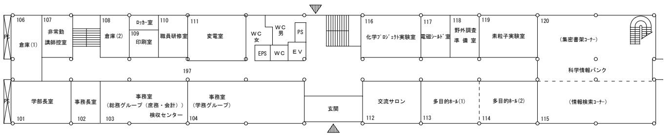
理学部A棟 1階平面図
