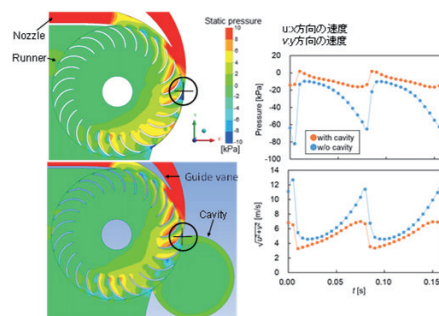
開発した新型水車（上）とコンピュータシミュレーションの結果例（下） [国内外3大学、2企業との連携研究開発]
