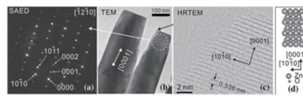
本研究室で創出したナノ材料の様々な構造
