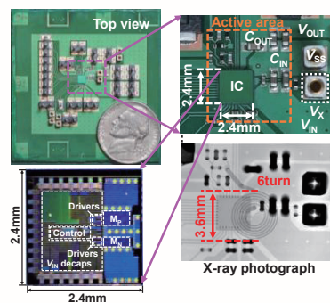
三次元集積実装したDCDC降圧コンバータ
