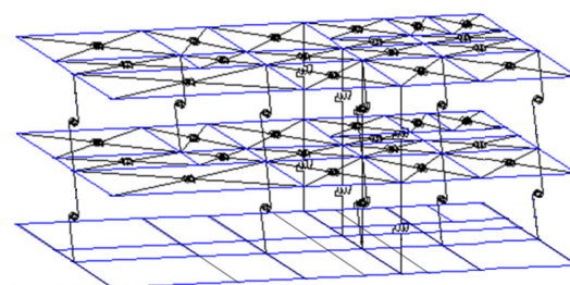
構造解析モデルによる耐震性能の検証
