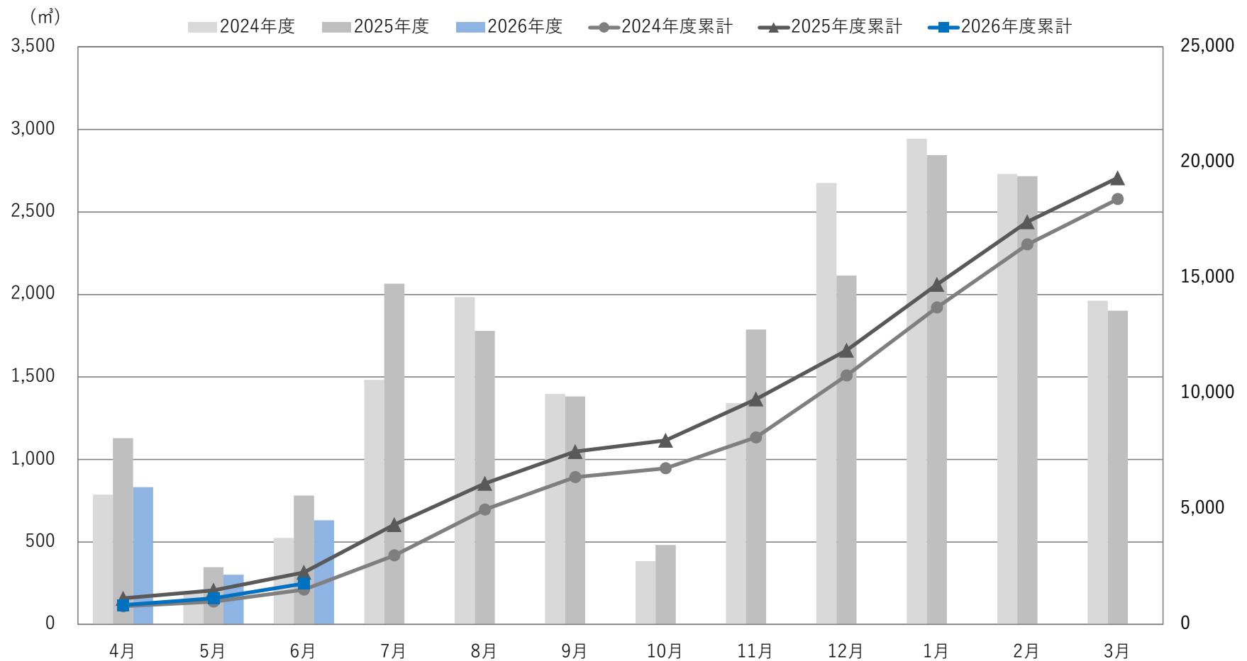
医学部保健学科中校舎 月別都市ガス使用量
