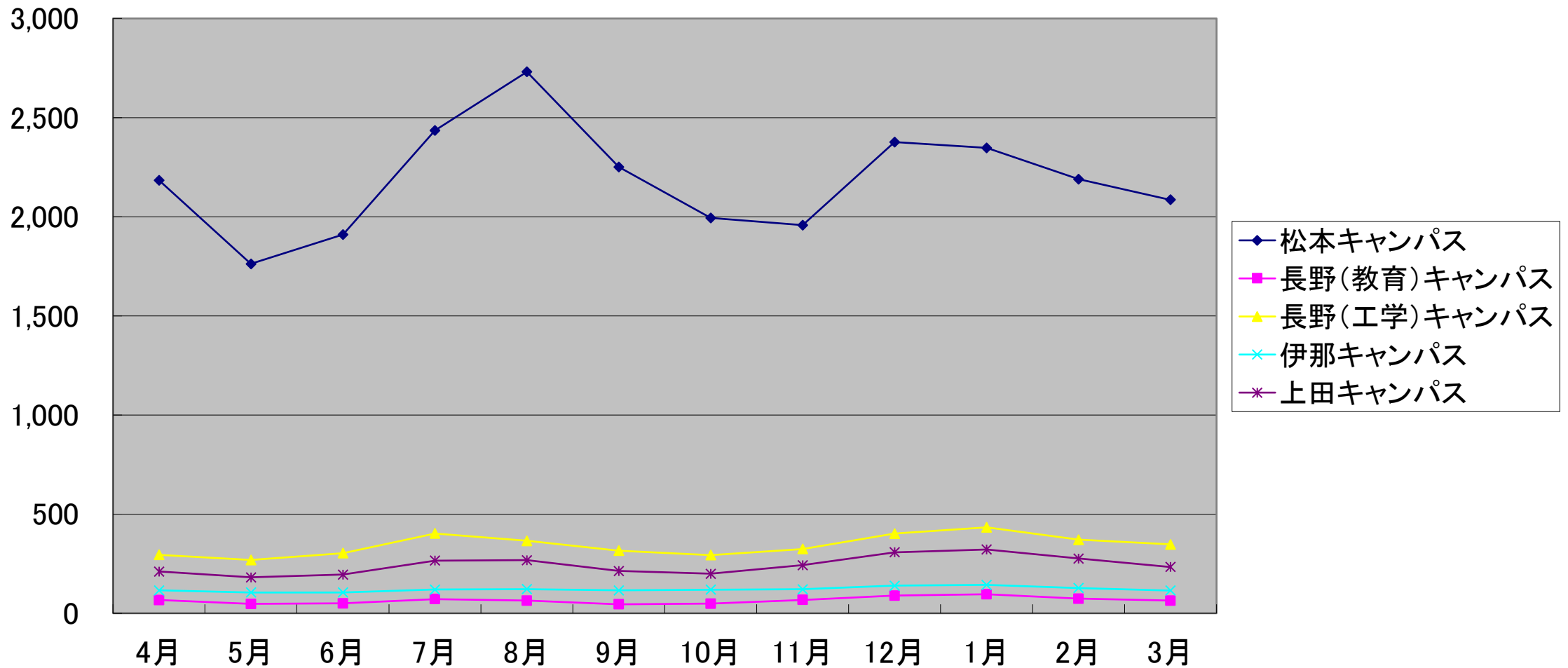
月別CO 2 排出量
