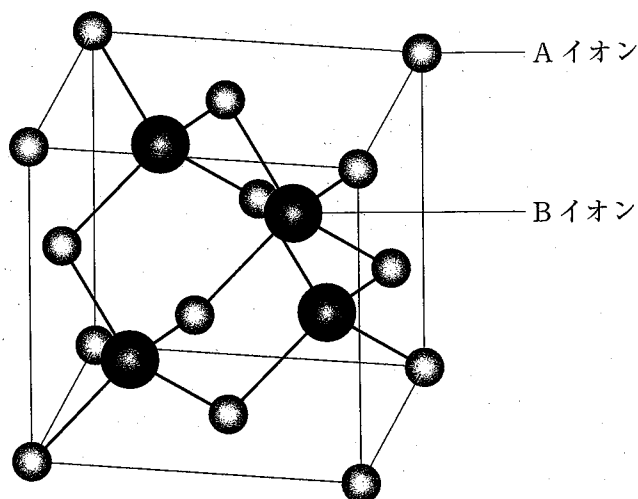
図 1 硫化亜鉛型結晶 AB の単位格子 (A：金属元素，B：非金属元素)
