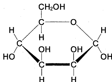
図3 \alpha -マンノースの構造式 太線は結合が手前にあることを示す。
