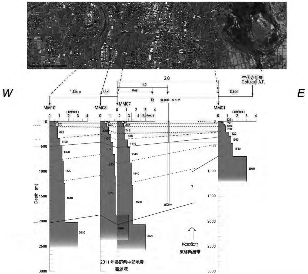
図 4.5 解析 S 波速度構造図
