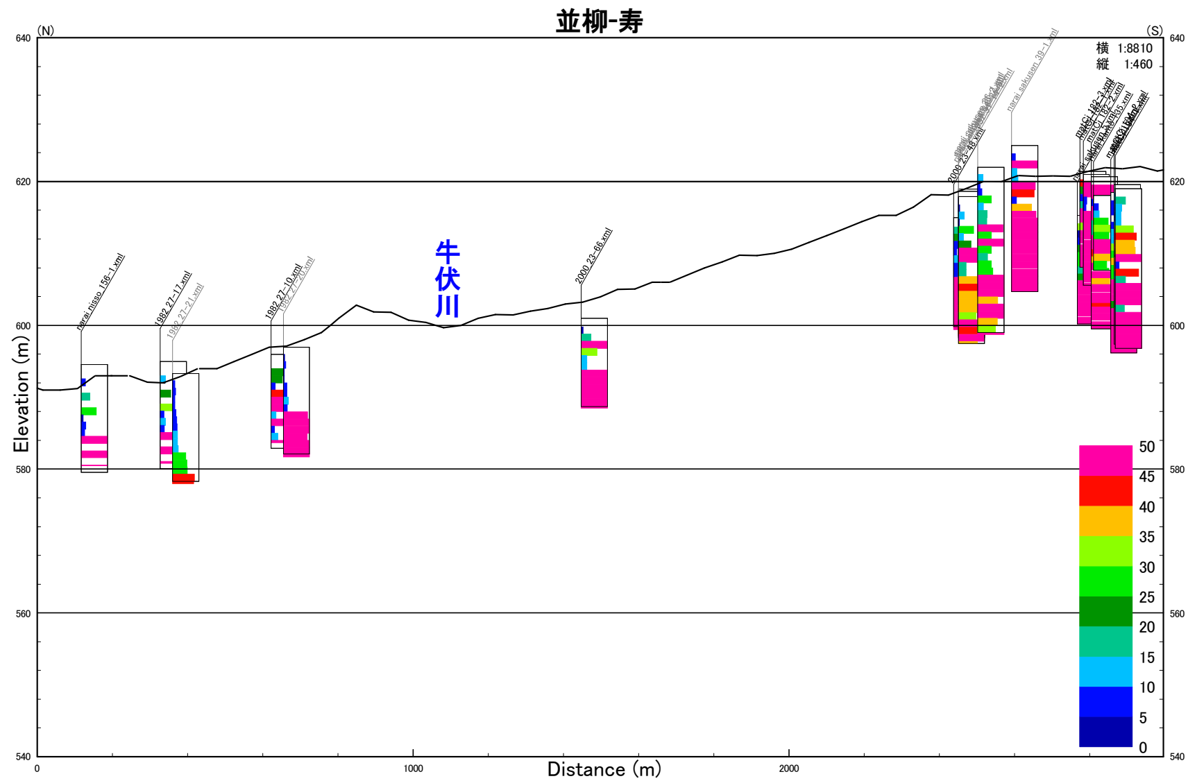
図 4-2-2 並柳-寿 線のボーリング柱状図 2 (N 値区分)
