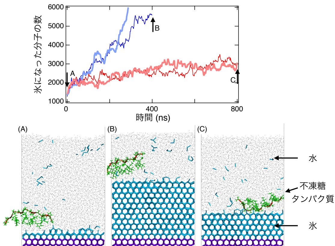
図3 成長する氷表面での不凍糖タンパク質の振る舞いをシミュレーションした図。上のグラフは不凍糖タンパク質の氷表面での向きが変わることで、氷の成長がどのように変化するかを時系列的に示したもの。横軸は時間経過を示しており、赤いラインを見ると氷の成長が止まっていることが分かる。この時、図Cのように、不凍糖タンパク質は疎水部分で吸着している。一方、青いラインのように、氷の成長が止まらない場合は、不凍糖タンパク質の親水部分が氷側を向いており、氷に吸着しない(図A,B)。
