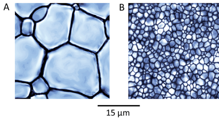
図 1: 不凍糖タンパク質がない場合(A)とある場合(B)による氷の成長の違い。A では大きな氷ができているが、B では小さいままで成長が止まっている。
