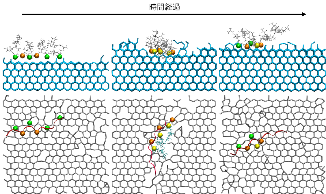
図 4 不凍糖タンパク質が氷の上を動く様子、上段は横から見た図、下段は上から見た様子。氷に吸着している疎水基を球体で表している。
