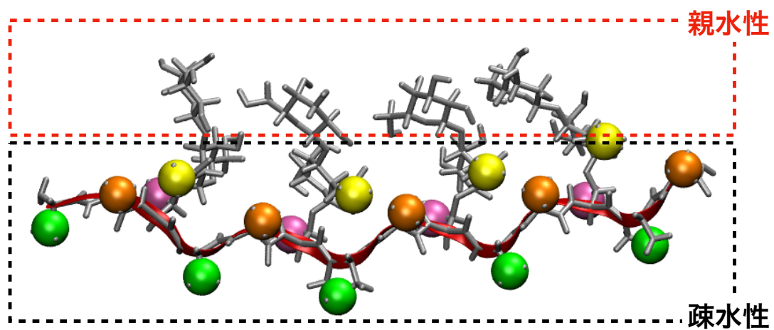
図 2 不凍糖タンパク質の水中での分子構造
