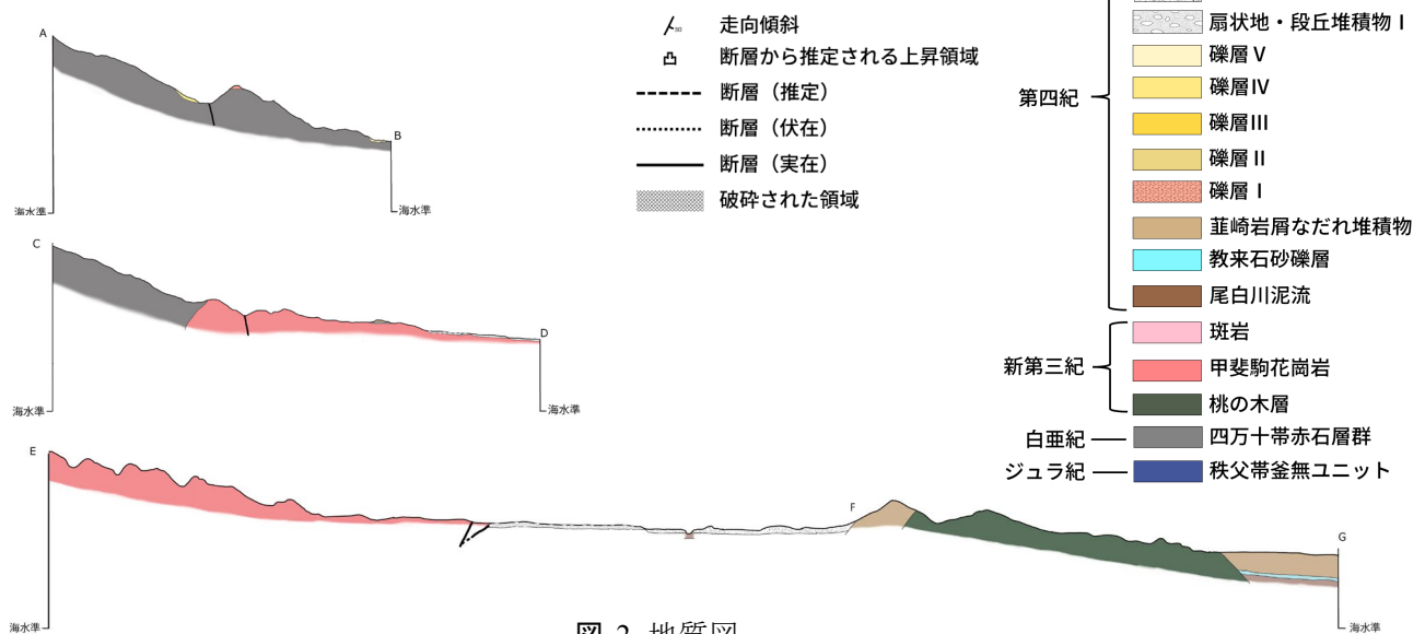
図-2 地質図
