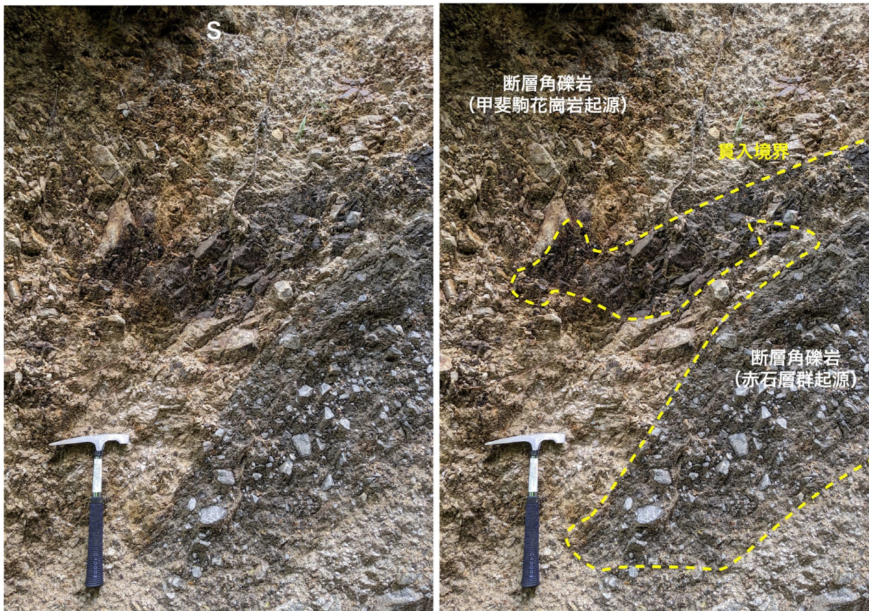
図-18 断層により破碎を受ける甲斐駒花崗岩と赤石層群の貫入境界 (Loc.4, 図-2)
