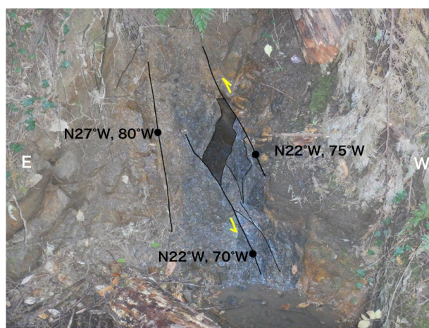
図-22 桃の木層中に認められる断層 (Loc.8, 図-2)
