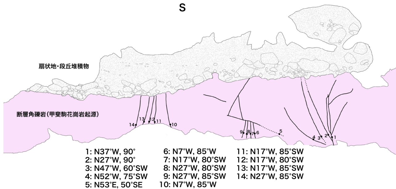
図-21 甲斐駒花崗岩中に認められる複数の断層 (Loc.7, 図-2)
