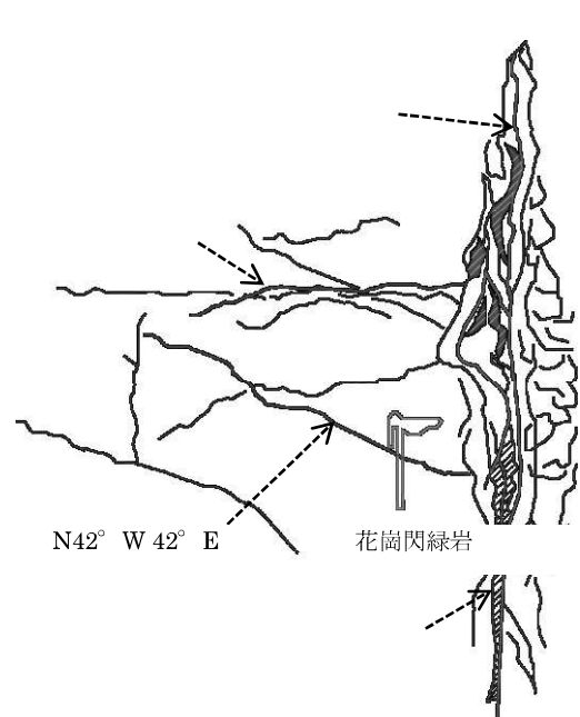
図-14 崖の湯断層群構成断層 塩沢川中流域
