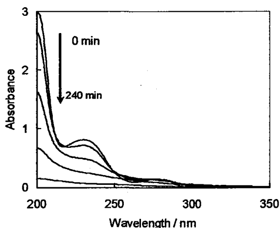
図 2 水中におけるフタル酸ジメチルのキセノン光照射にともなう UV-Vis 吸収スペクトルの変化
