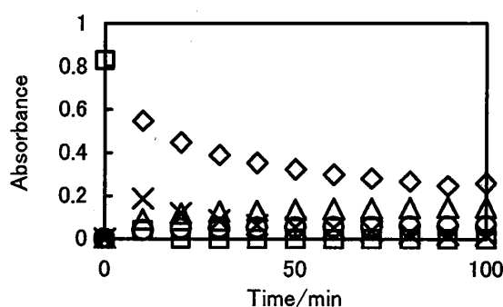
図5 気相のトリクロロエチレンへの光照射時間にもなう親分子と生成物の吸光度の変化：トリクロロエチレン(□)、DCAC(x)、 \text{COCl}_2 (◇)、HCl(△)、CO(○)
