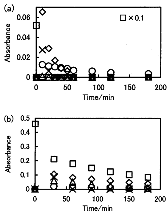
図6 (a)アロフェンまたは(b)石炭灰と共存下における気相のトリクロロエチレンへの光照射時間にもなう親分子と生成物の吸光度の変化：トリクロロエチレン(□)、DCAC(x)、 \text{COCl}_2 (◇)、HCl(△)、CO(○)
