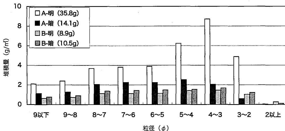
図2 地点Aと地点Bにおける明暗条件による浮遊土砂堆積量の粒度分布。
