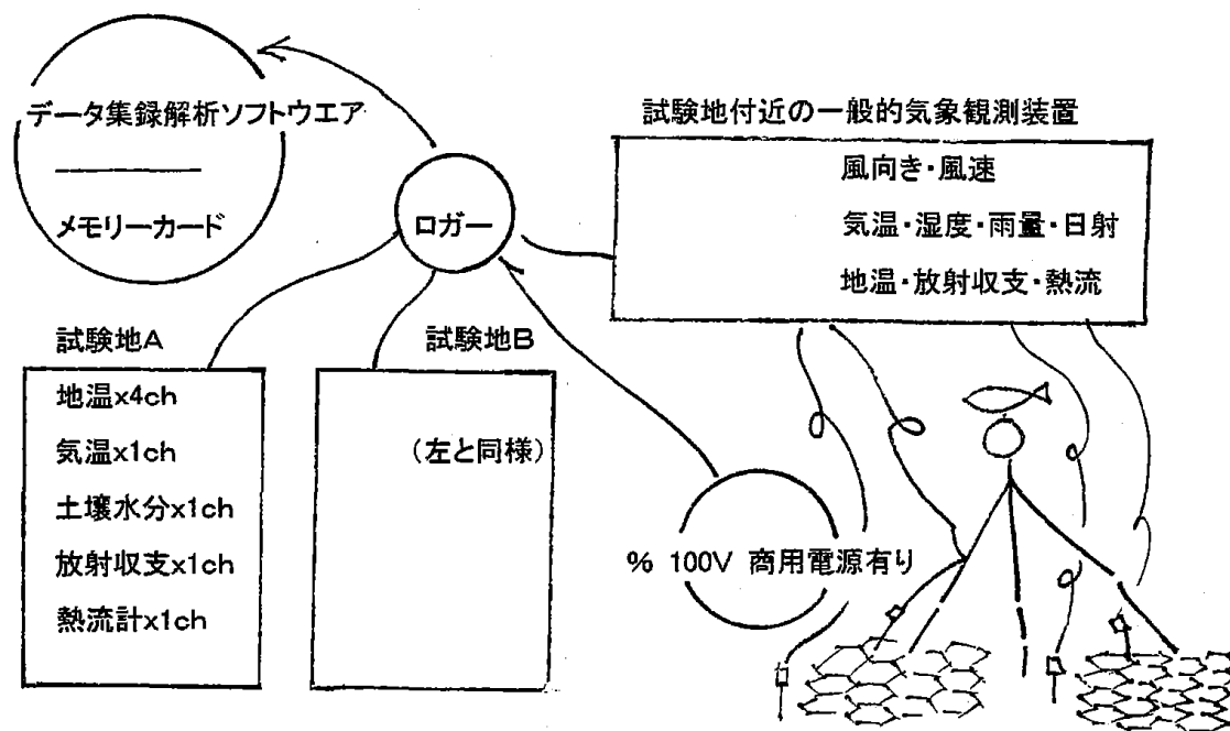
図 1. 測定機器配置と測定項目の概略
