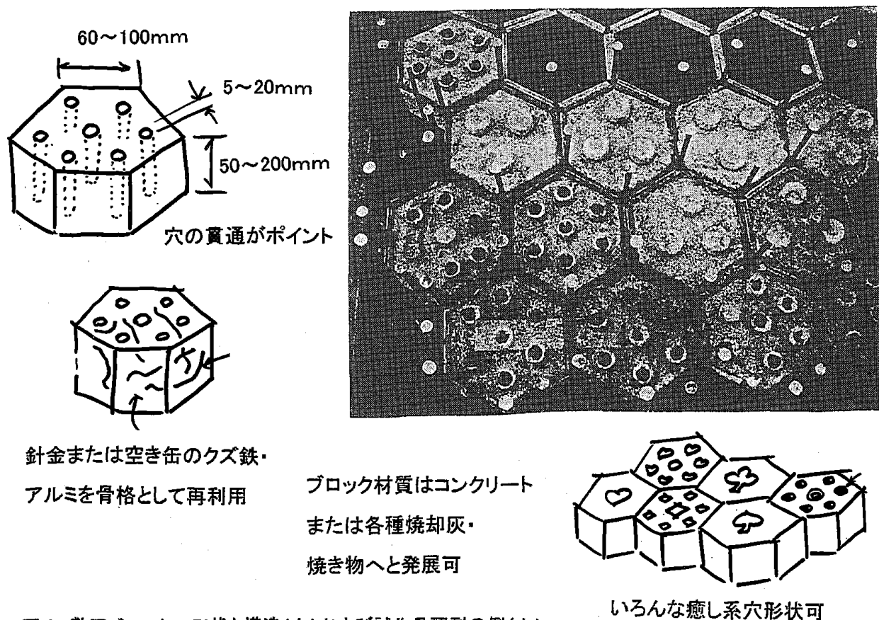
図 2. 敷石ブロックの形状と構造(左)および試作品配列の例(右)
