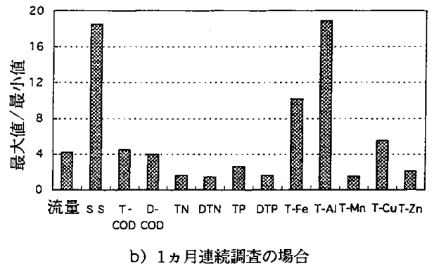
図-10 流量および各成分濃度の最小値と最大値の比(2)
