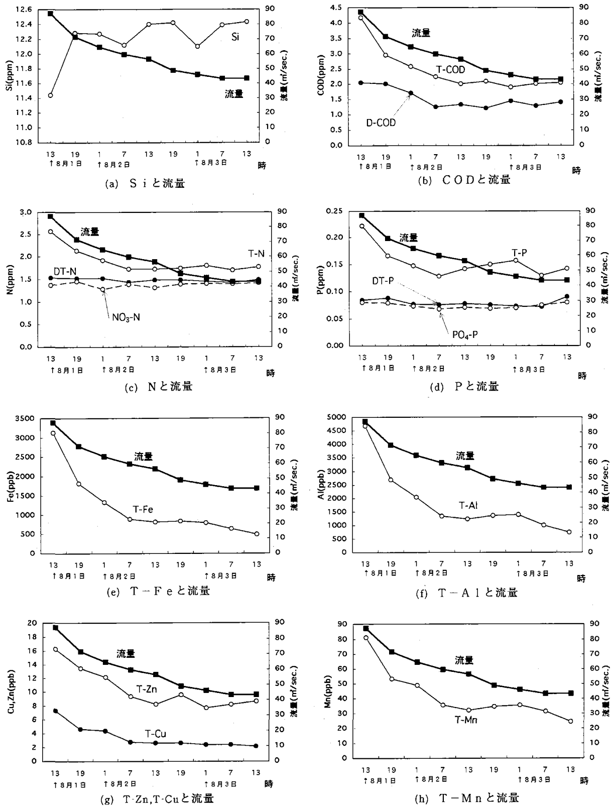
図-6 48時間連続調査における古舟橋地点の流量と水質の変化傾向(2) (Si, COD, N, P, Al, Cu, Zn, Mn)
