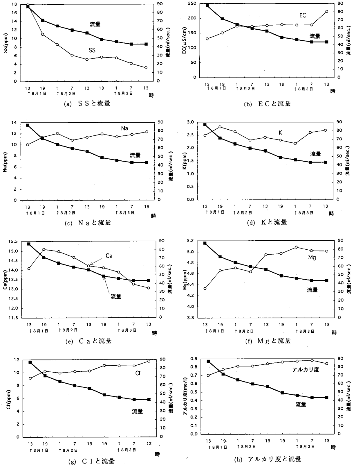
図-5 48時間連続調査における古舟橋地点の流量と水質の変化傾向(1) (SS, ES, Na, K, Ca, Mg, Cl, アルカリ度)
