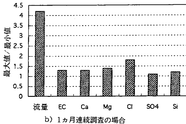
図-9 流量および各成分濃度の最小値と最大値の比(1)
