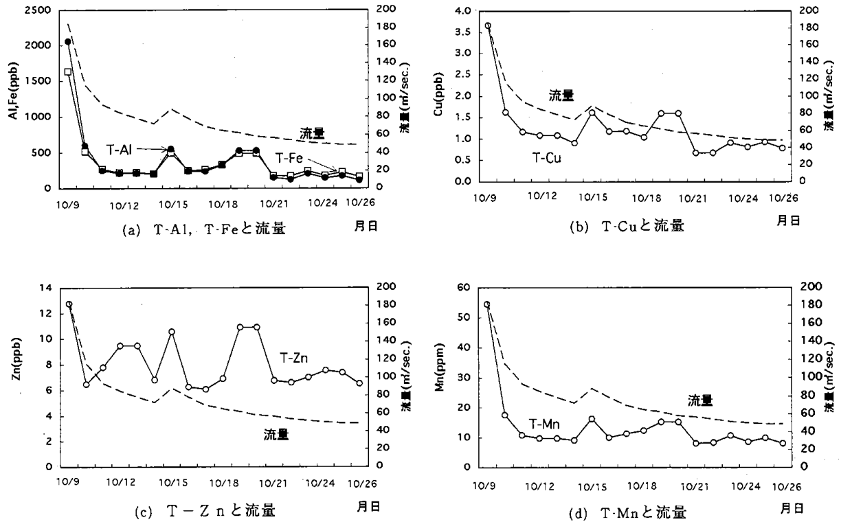
図-8 1ヵ月連続調査における流量と水質の変化傾向(2) (Fe, Al, Cu, Zn, , Mn)
