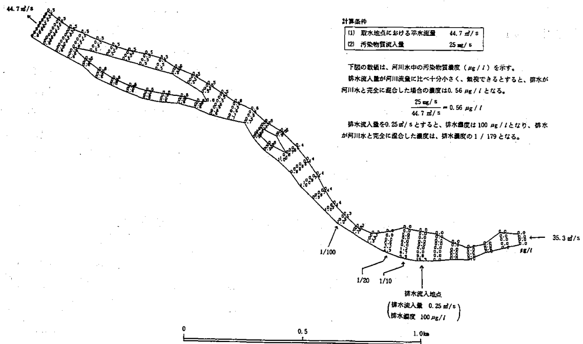
図-1 汚染物質濃度の分布 (A-1)
