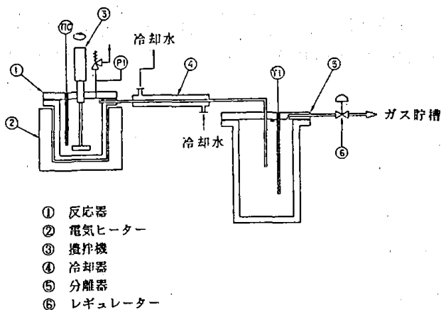
図2 汚泥油化および高压蒸留実験装置 7)
