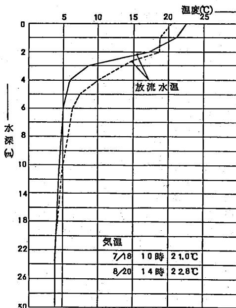
図4. 貯水池の水温分布の実例
