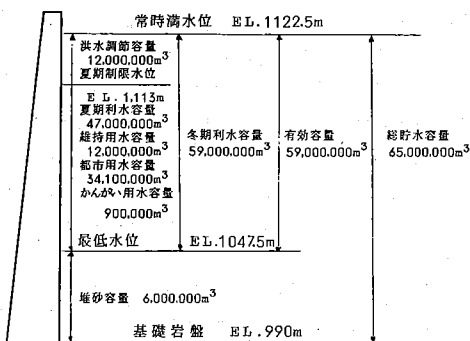
図3. 貯水池容量配分図
