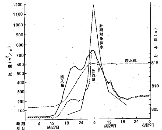
図2. 天竜川・美和ダムにおける昭和36年6月28日洪水
