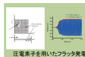
圧電素子を用いたフラッタ発電
